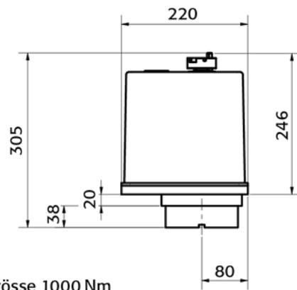
Abbildung: Variante Standardgrösse 1000 Nm Illustration : variante dimension standard 1000 Nm Figura: Variante dimensioni standard 1000 Nm
